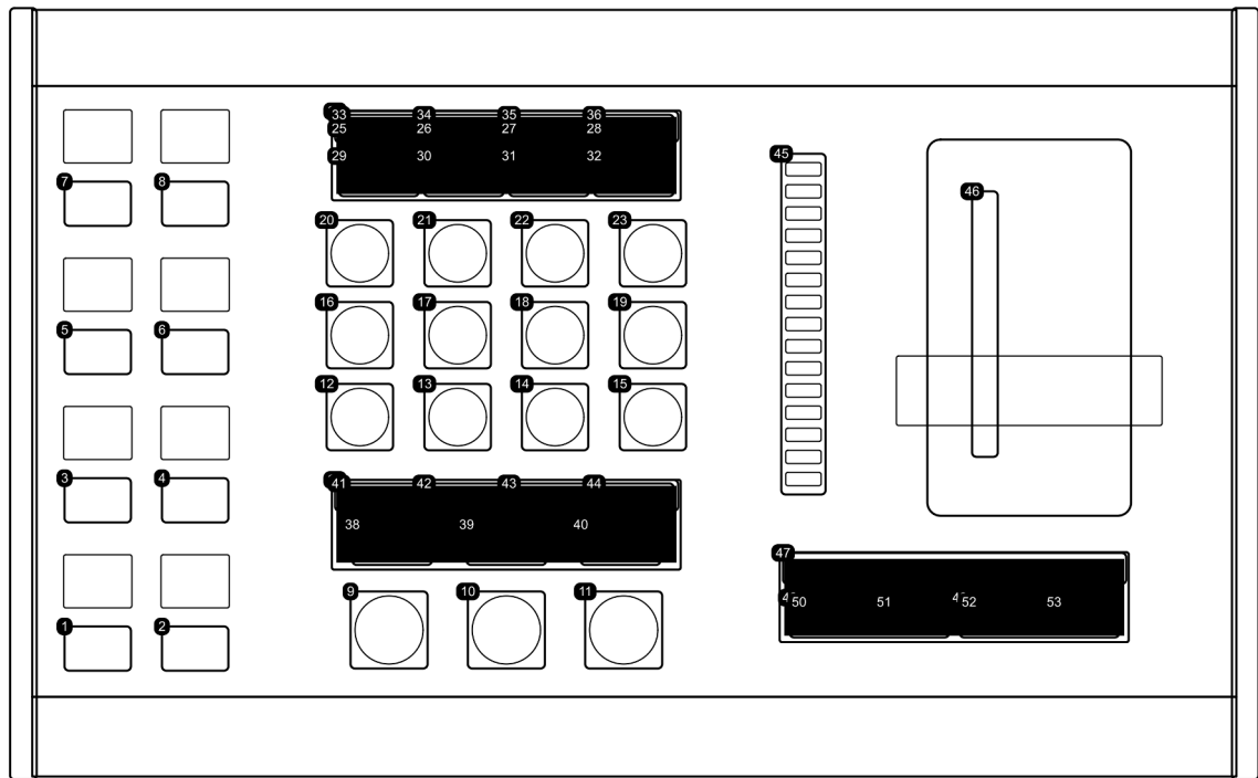
Figure 2: T-Block Right のハードウェアコンポーネント図 (コンポーネント ID (HWc ID) 付き)
