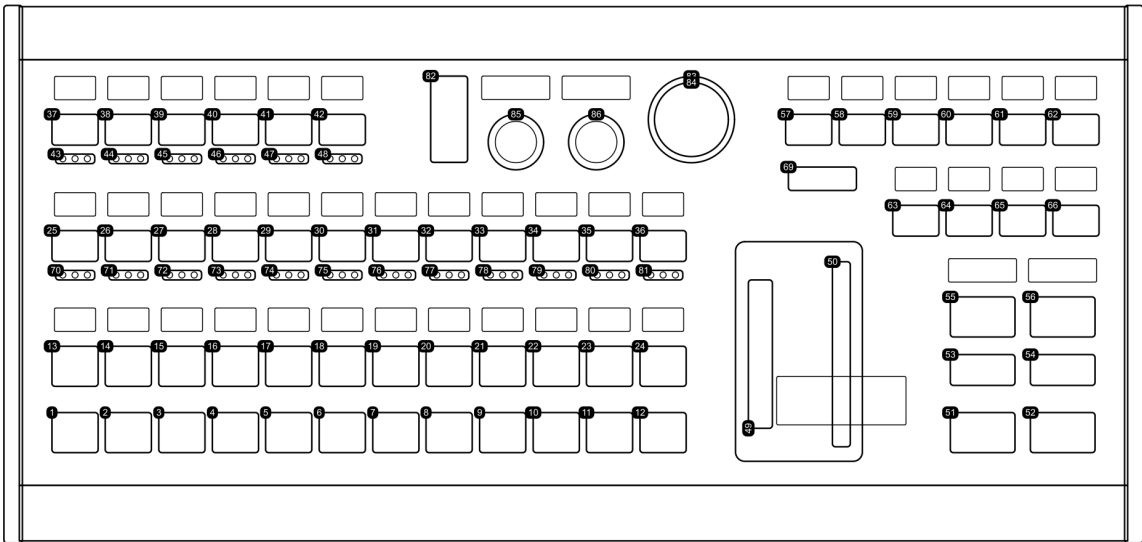
Figure 2: Air Fly Pro のハードウェアコンポーネント図 (コンポーネント ID (HWc ID) 付き)
